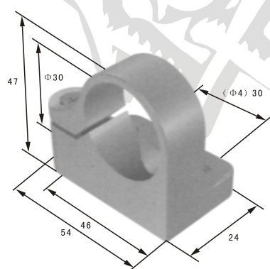
Φ30安装架
