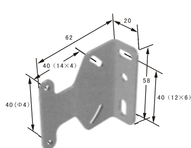
L50安装架
