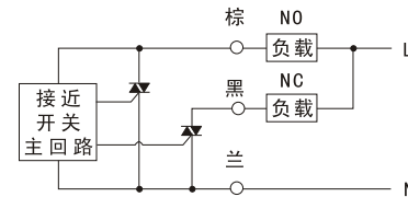
AC 三线NO+NC输出回路图(GT)
