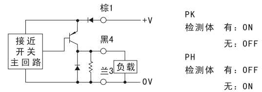
DC PNP型NO、NC输出回路图(PK、PH)
