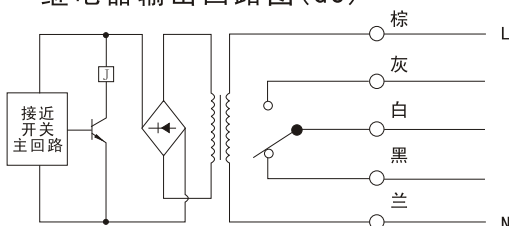
AC 继电器输出回路图(GJ)
