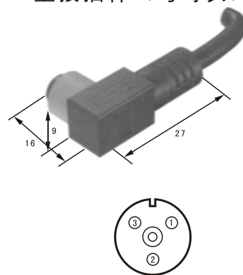
I型接插件（弯母头）
