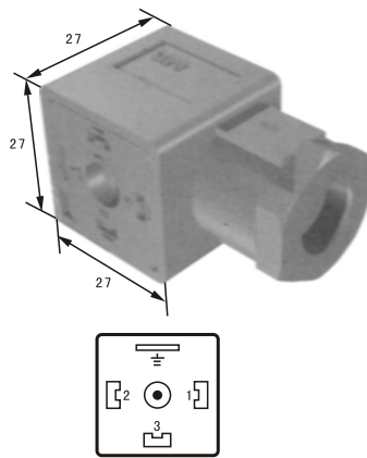
X型接插件
