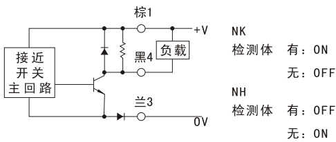
DC NPN型NO、NC输出回路图(NK、NH)
