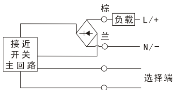
AC/DC 二线NO\NC可选输出回路图(GC/DC)
