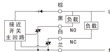
AC 四线NO+NC输出回路图(ST)
