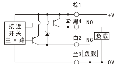
DC PNP型NO+NC输出回路图(PT)
